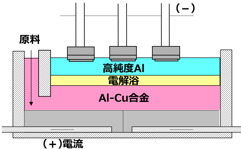
三層電解法
